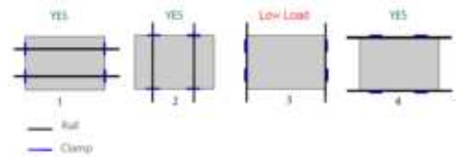
図 3. 架台の構成
