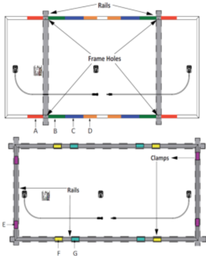
Figura 4: Zona de montaje para los módulos Performance
